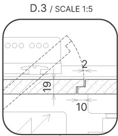
D.3 / SCALE 1:5
