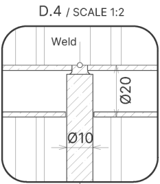
D.4 / SCALE 1:2
